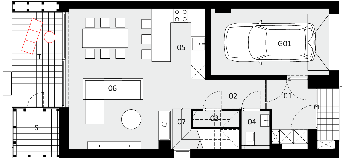
Rzut parteru
