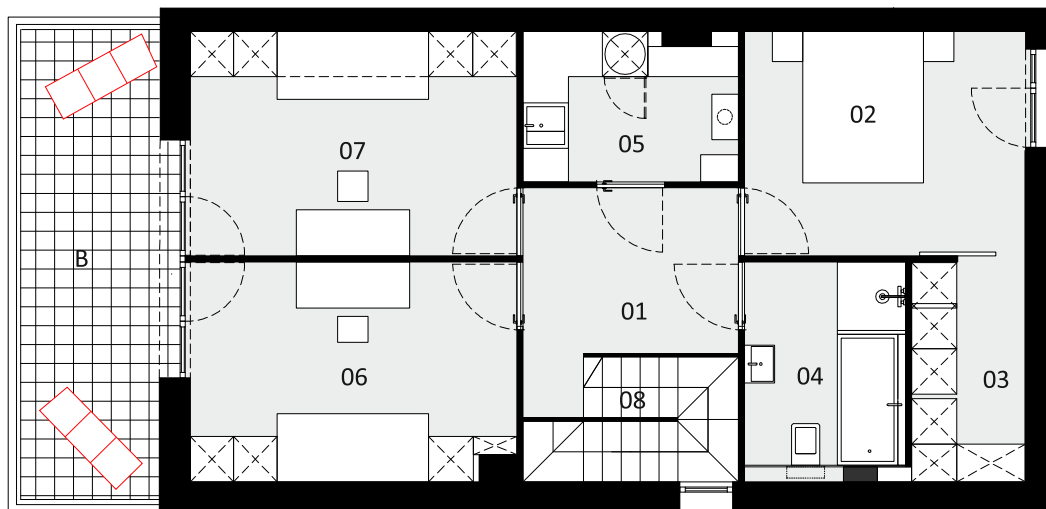
Rzut piętra
