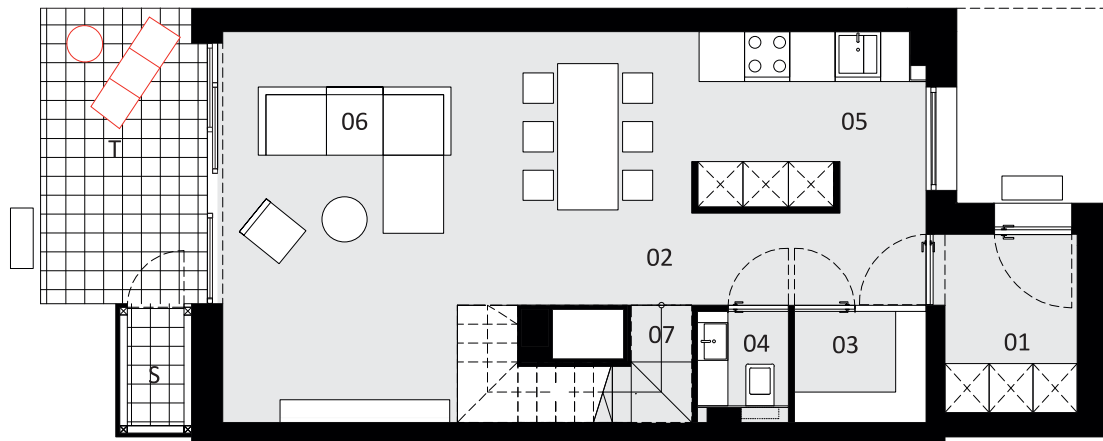
Rzut parteru
