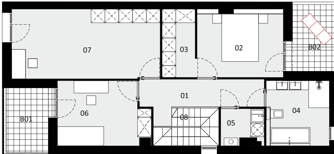
Rzut piętra
