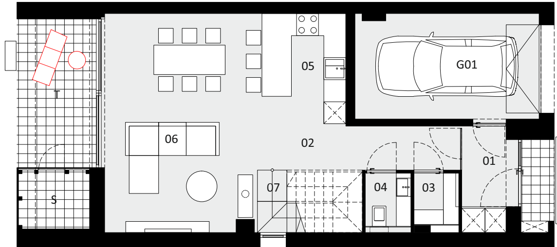
Rzut parteru
